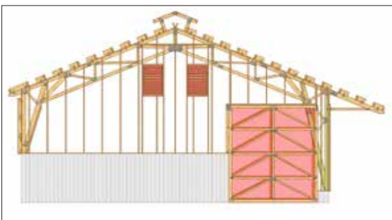
Gavlvegg med port
